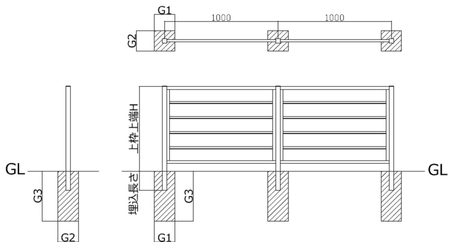
1型（120サイズ 隙間15mm）
