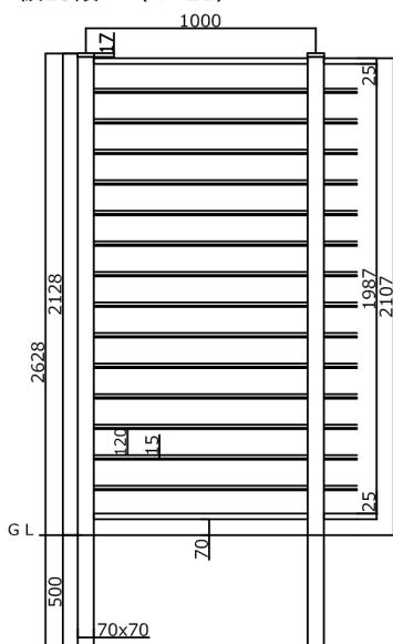
板15段 (T-21)
