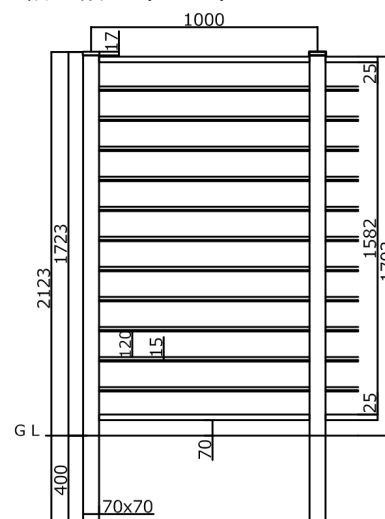
板12段 (T-17)
