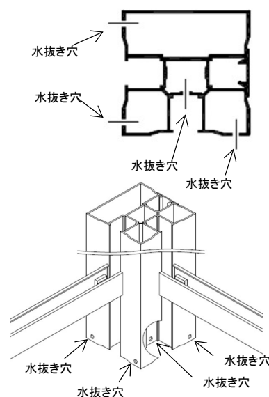
コーナー柱
