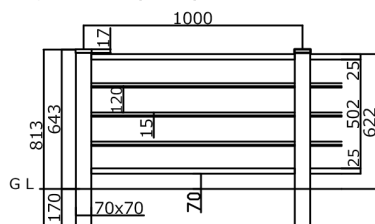
板4段 (T-6)
