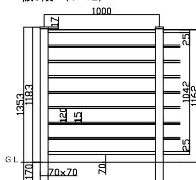
板8段 (T-12)
