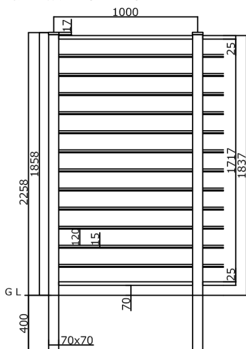
板13段 (T-18)
