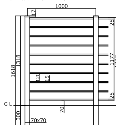
板9段 (T-13)
