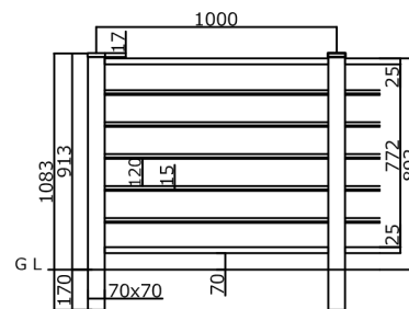
板6段 (T-9)
