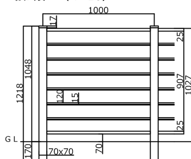
板7段 (T-10)
