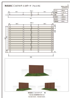
図面/パース
