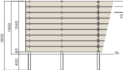
ニコボード 140サイズ 隙間10mm 板9段(T-14) 柱60×60
