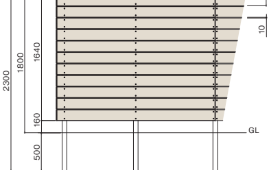
ニコボード 140サイズ 隙間10mm 板11段(T-18) 柱60×60
