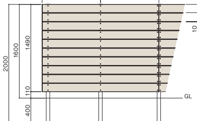
ニコボード 140サイズ 隙間10mm 板10段(T-16) 柱60×60
