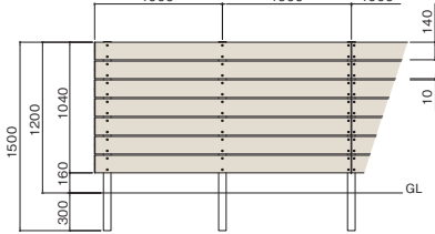
ニコボード 140サイズ 隙間10mm 板7段(T-12) 柱60×30
