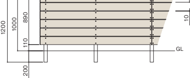
ニコボード 140サイズ 隙間10mm 板9段(T-14) 柱60×60
