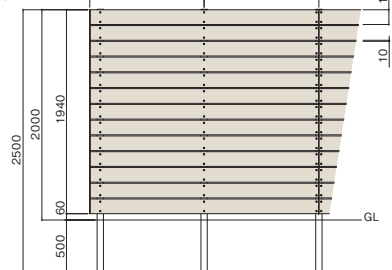
ニコボード 140サイズ 隙間10mm 板13段(T-20) 柱60×60
